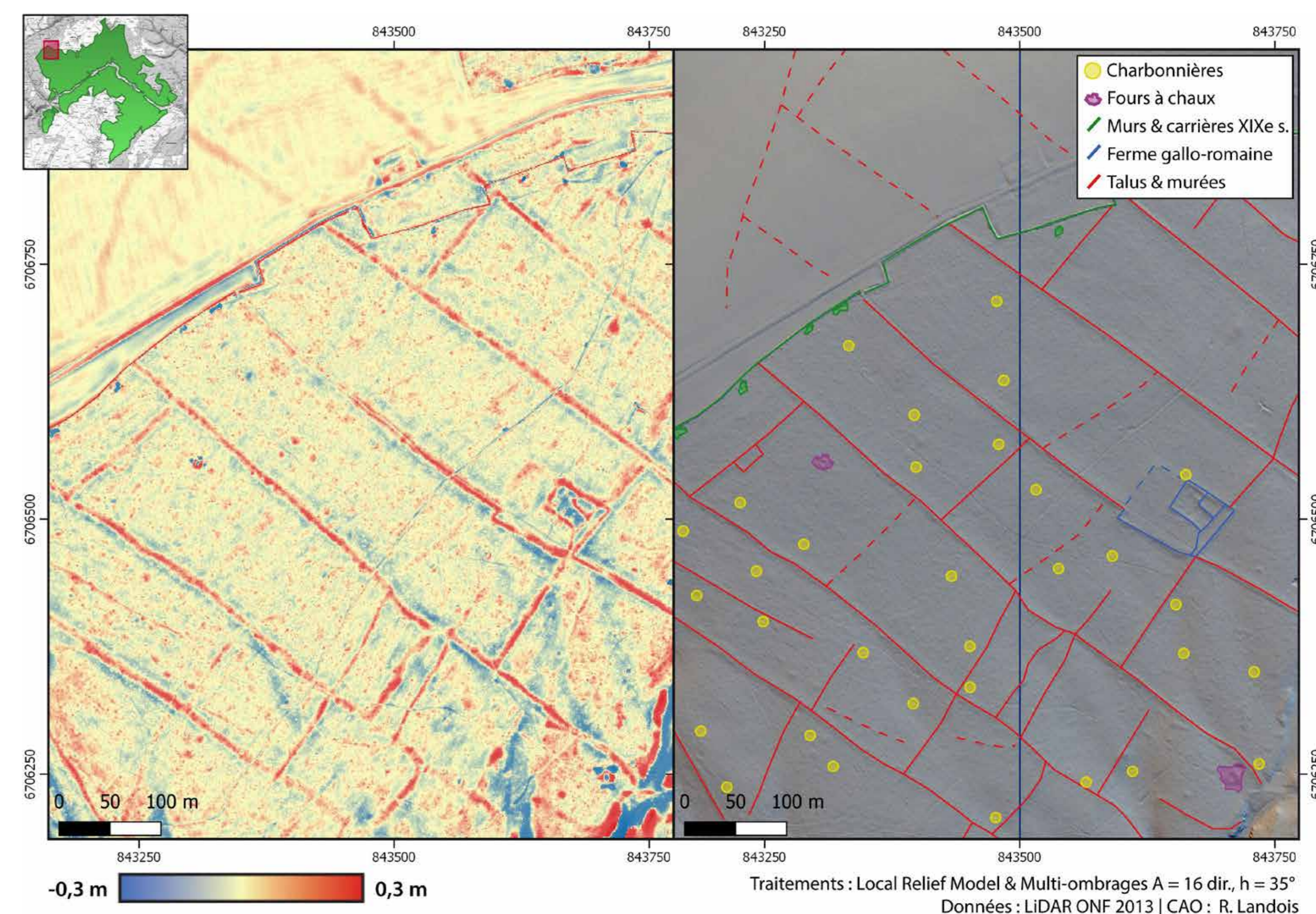
Extrait et interprétation des données LiDAR au lieu-dit « les Fouillies » (commune de Val-Suzon, Côte-d'Or).
