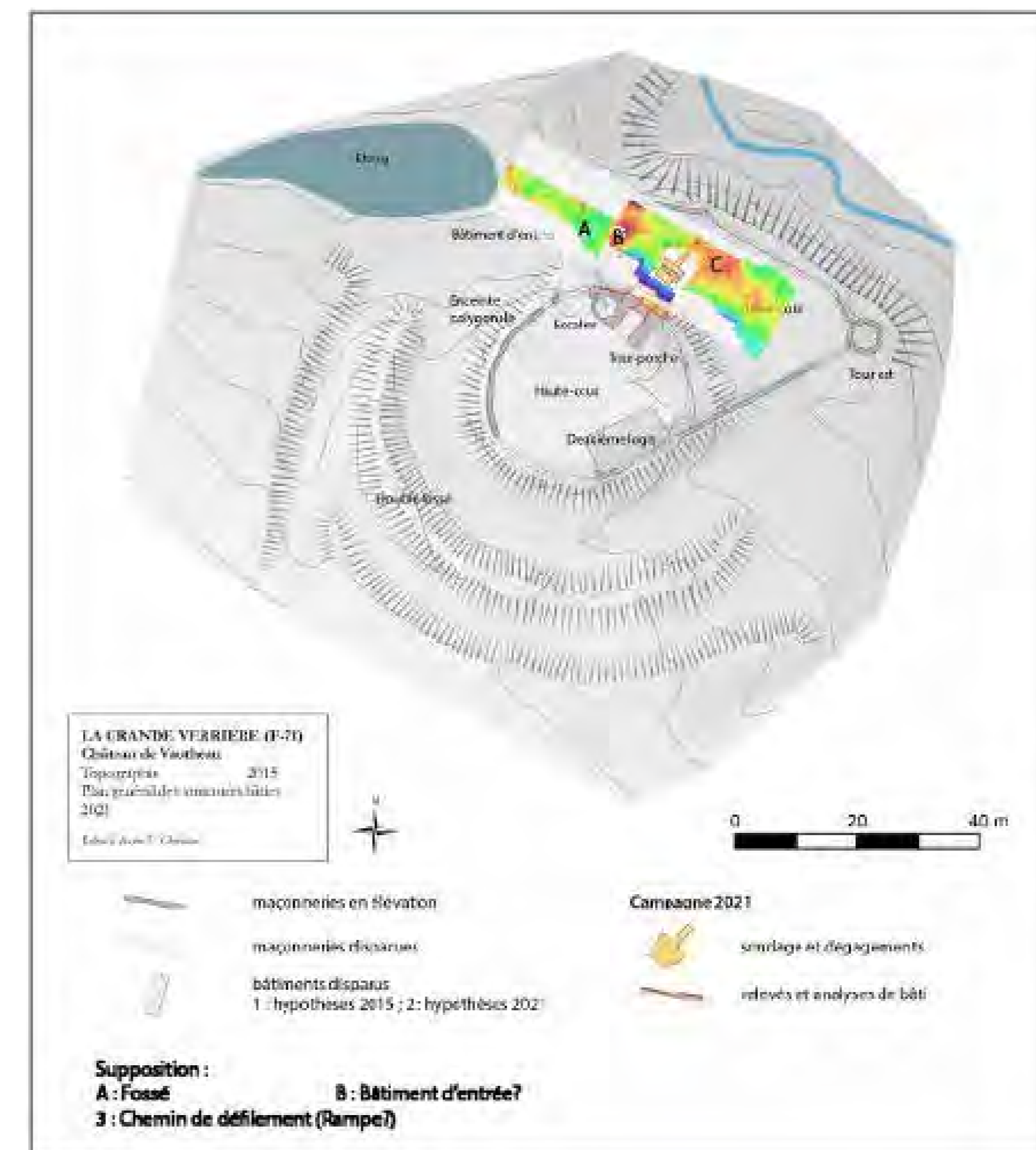
Résultat de la prospection électrique de M. Mignot.
